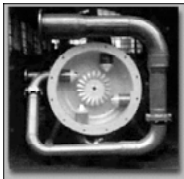
Turbina Pelton a 4 getti da 100 kW (Fonte: Tamanini)
