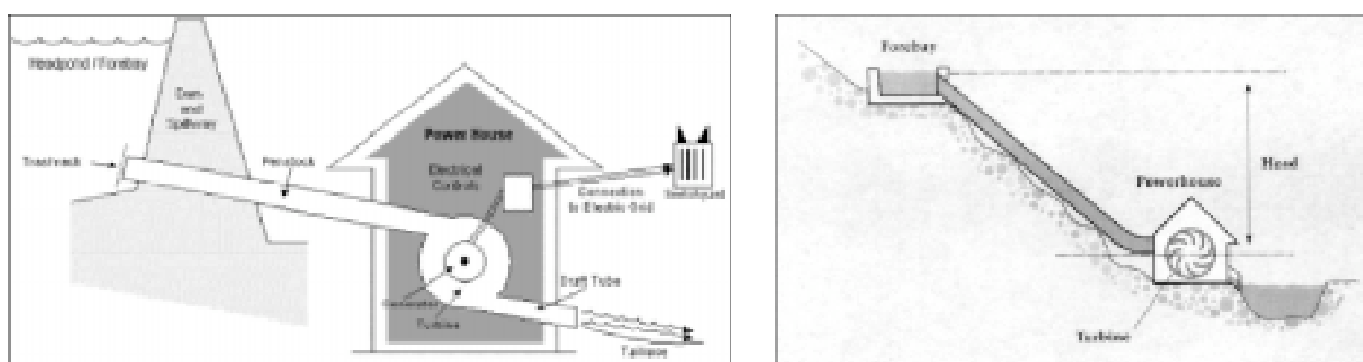
Schema di dettaglio (camera di carico, condotta, centrale, restituzione in alveo)
