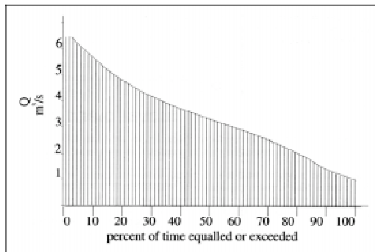
Curva di durata delle portate
